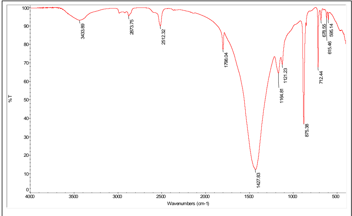
图 3: 灼烧残余的 FTIR 谱图
