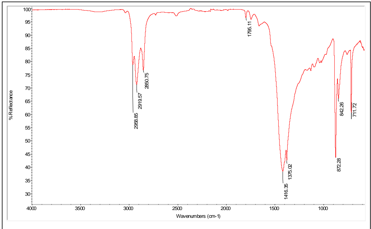
图 1: 原样的 FTIR 谱图-黑色部位
