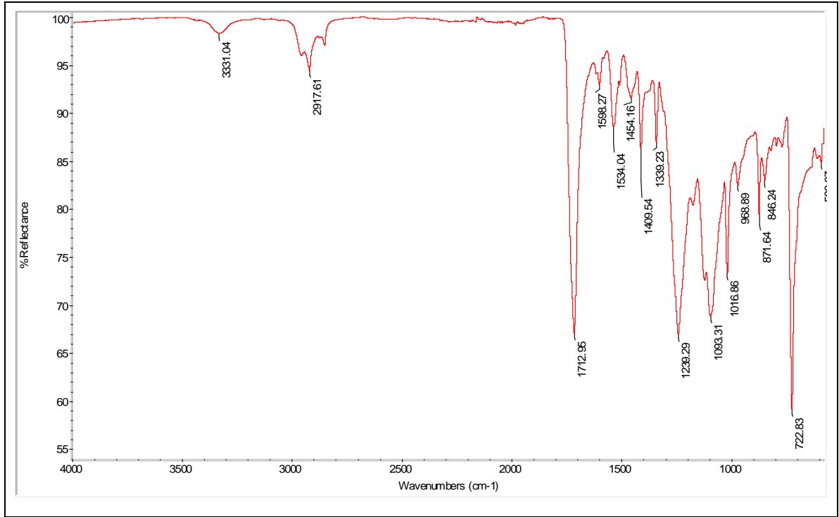
图 2: 原样的 FTIR 谱图-白色部位
